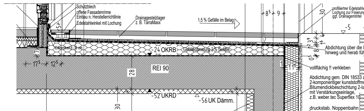
Ausschnitt A2 M 1 : 5
